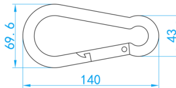
AISI316 Carabiner
